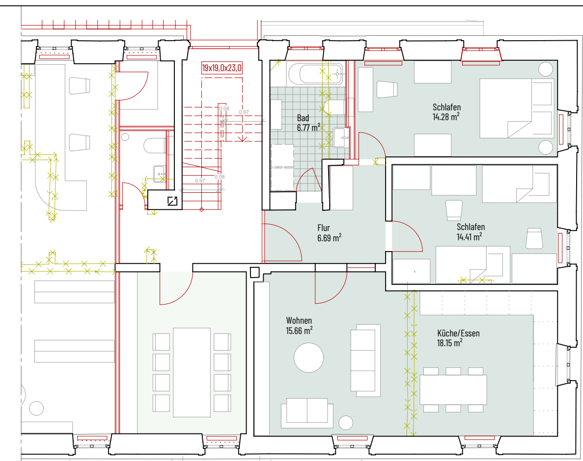
Alternative Wohnung 1 M 1:100
