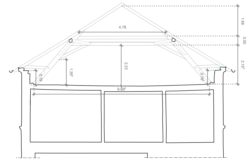
Querschnitt Dachstuhl Bestand M 1:100
